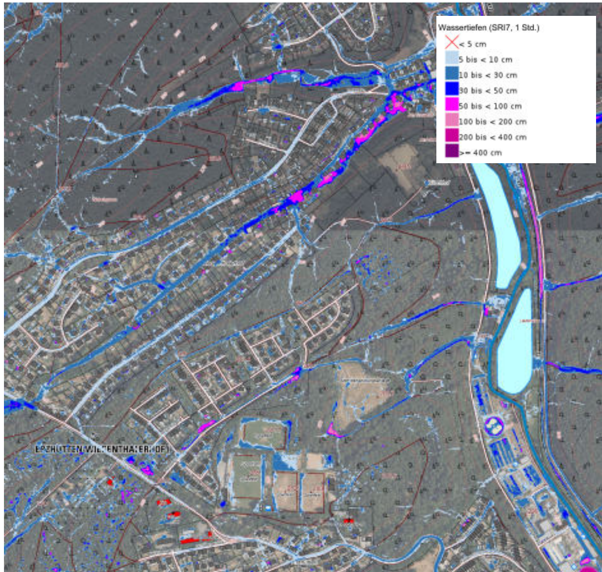
Abbildung 09: Ausschnitt Sturzflutgefährdungskarten SRI 7 (MKUEM, 2025) für Gebiet der Oberen Lauter
