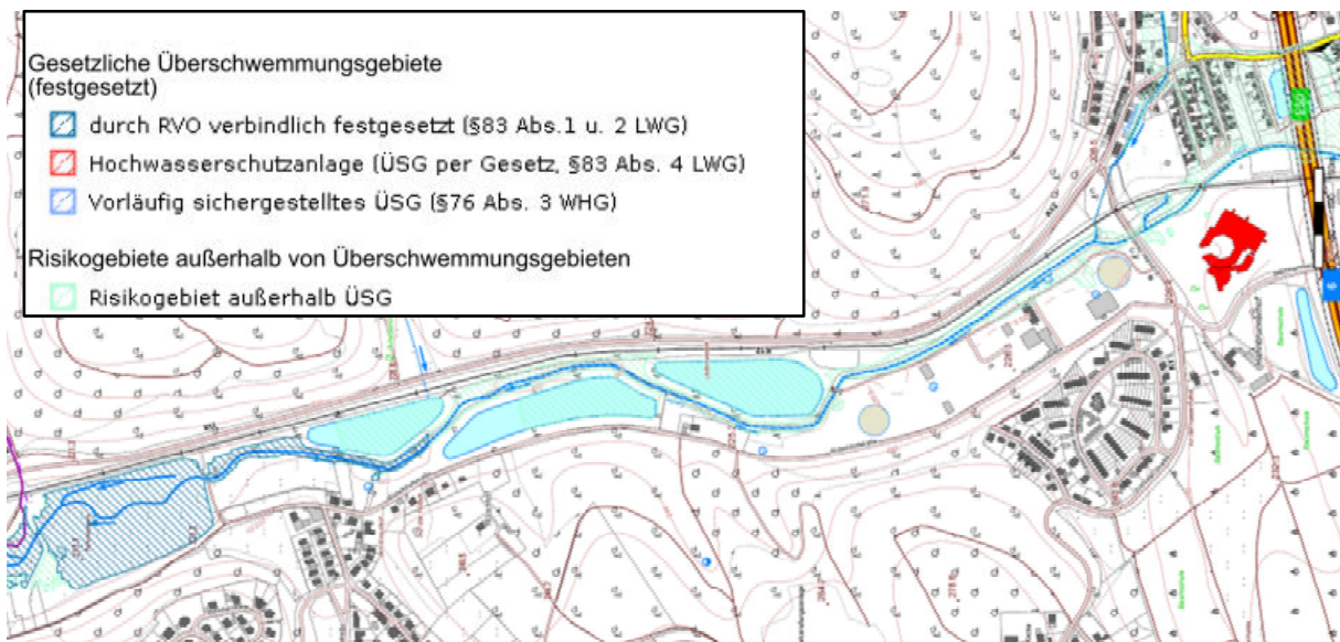
Abbildung 12: Überschwemmungs- und Risikogebiete an der Lauter (MKUEM, 2025)
