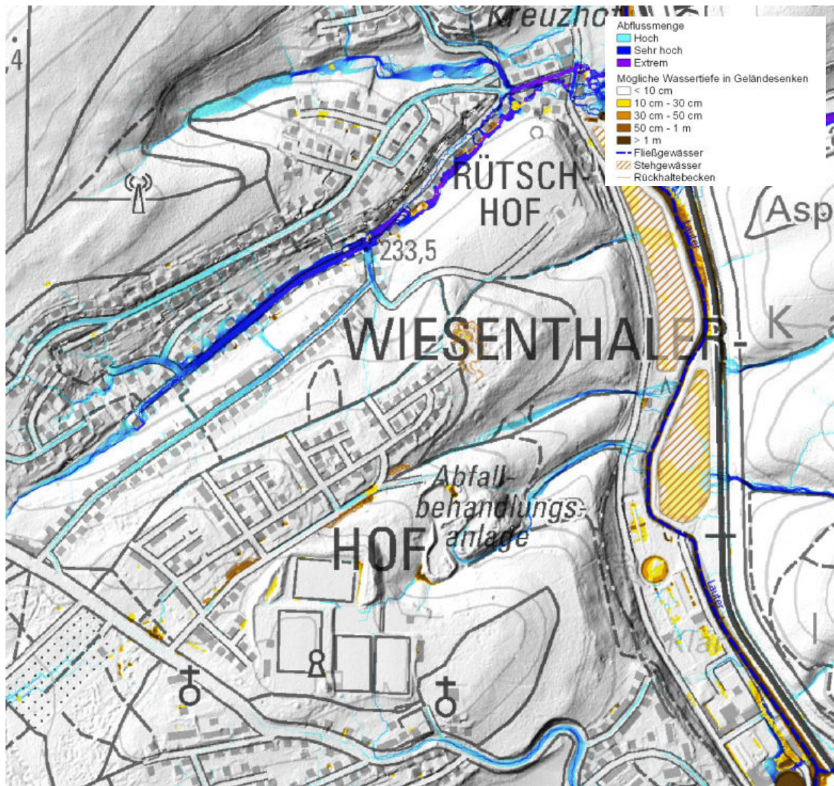
Abbildung 10: Ausschnitt Starkregengefahrenkarte SRI 7 (STE, 2022) für das Gebiet der Oberen Lauter
