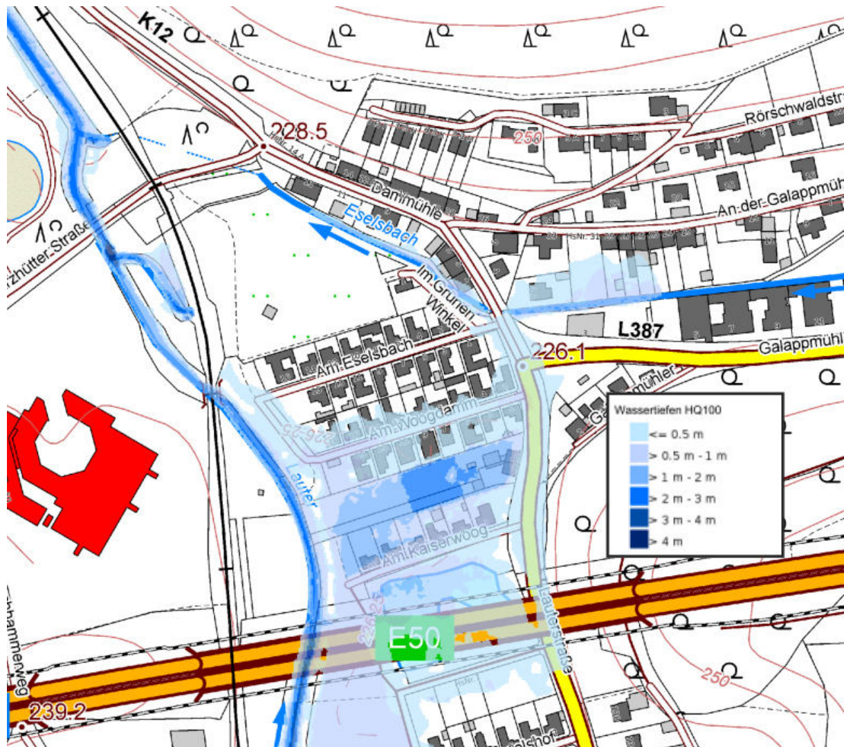
Abbildung 13: Wassertiefen HQ100 im vorläufigen ÜSG der Lauter (MKUEM, 2025)
