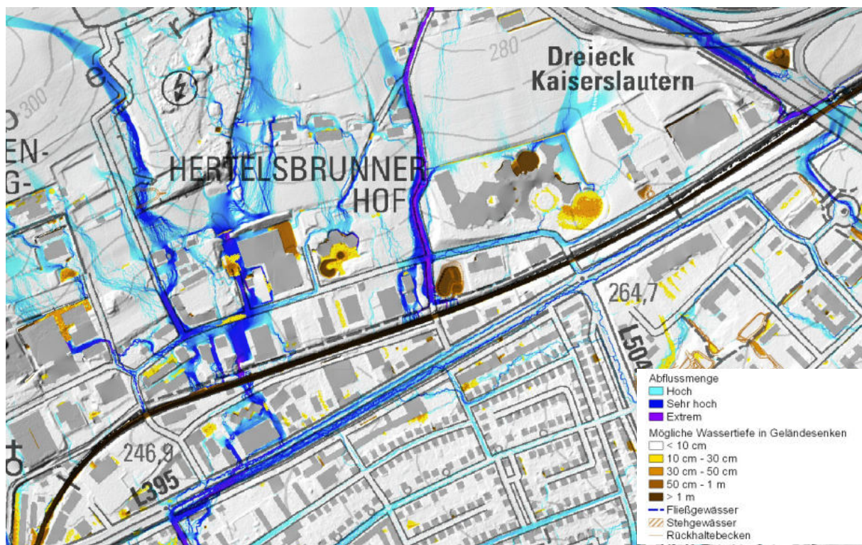
Abbildung 12: Ausschnitt Starkregengefahrenkarte SRI 7 (STE, 2022) für das nördliche Stadtgebiet
