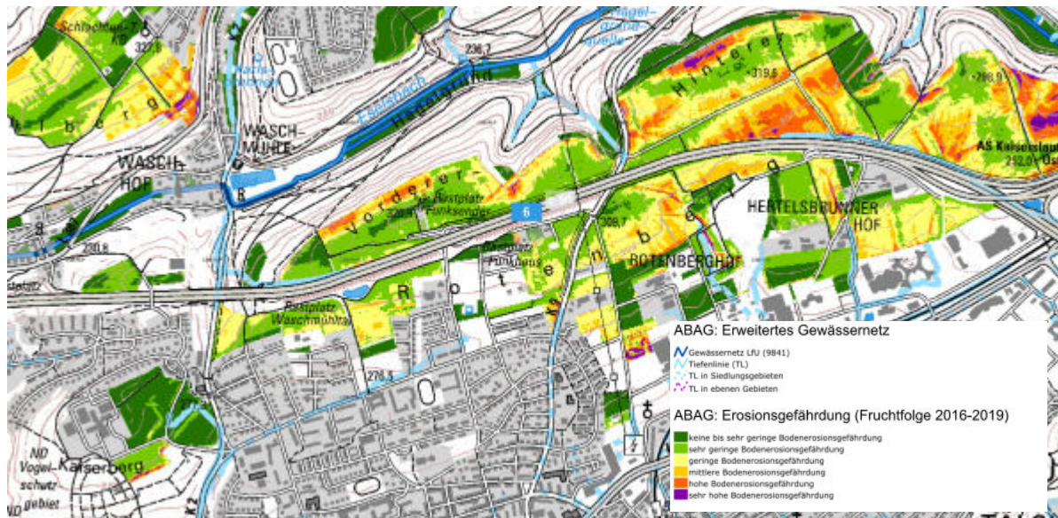
Abbildung 10: Erosionsgefährdung BG 6 gemäß ABAG (Landesamt für Geologie und Bergbau RLP, 2025)
