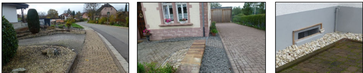
Abbildung 08: Beispiele von Objektschutzmaßnahmen (Überbogen, Geländemodellierungen, Aufkantung am Kellerfenster)
