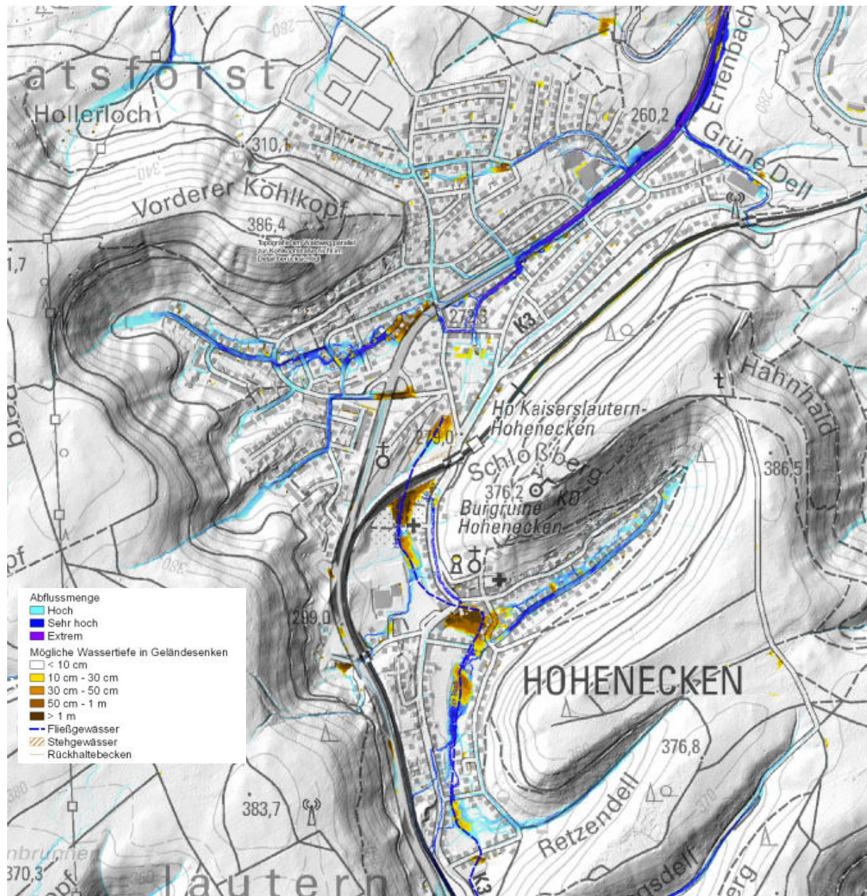
Abbildung 11: Ausschnitt Starkregengefahrenkarte SRI 7 (STE, 2022) für Hohenneck
