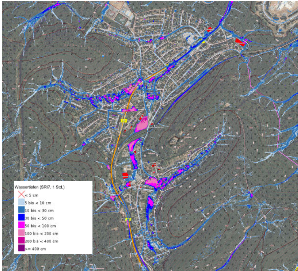
Abbildung 09: Ausschnitt Sturzflutgefährdungskarten SRI 7 (MKUEM, 2024) für Hohenecken
